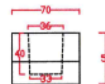
sec A-A
